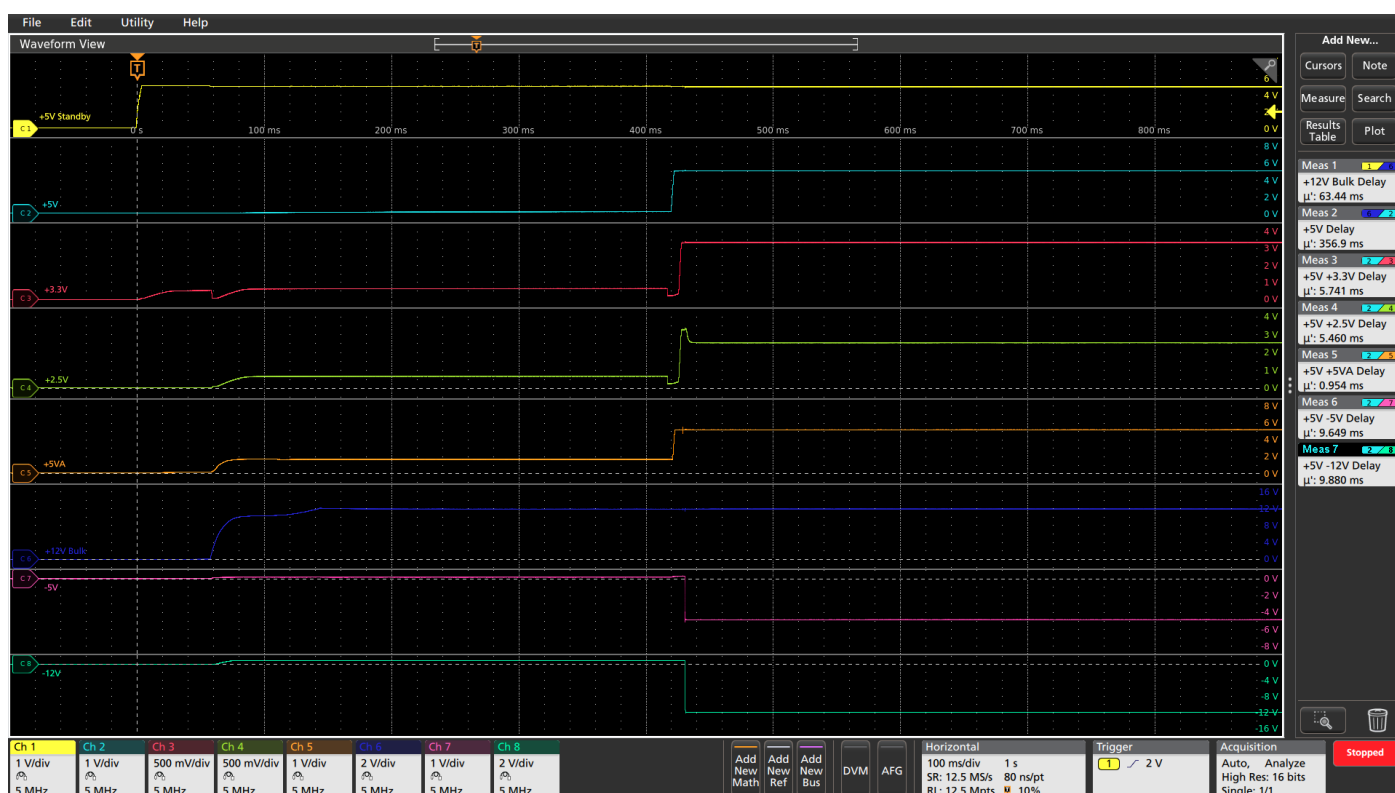
Использование автоматических измерений позволяет получить характеристики источника электропитания.
