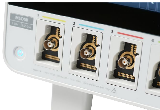
Технология FlexChannel обеспечивает максимальную гибкость. Каждый вход можно сконфигурировать как один аналоговый или восемь цифровых каналов в зависимости от типа подключаемого пробника.
